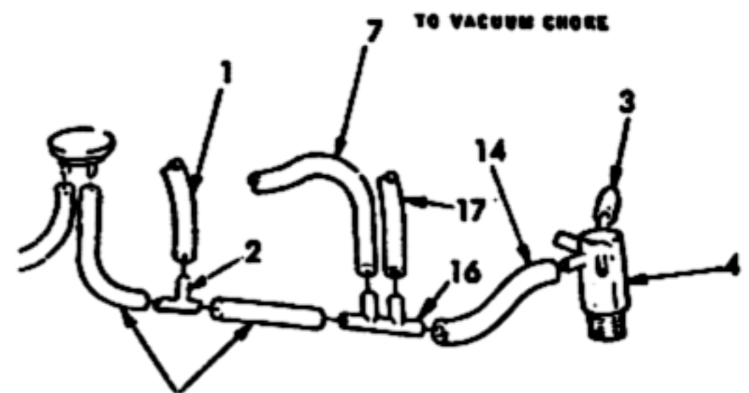
VIEW Y
